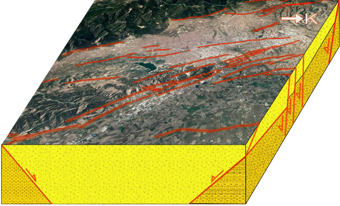
Şekil 5- Denizli'nin genel yeraltı yapısı. Kırmızı çizgiler diri fayları, Sarı noktalı alanlar alüvyon ve benzeri zayıf zeminler, koyu sarı alanlar ise nispeten dayanımlı genç gösel çökelleri göstermektedir (Ölçeksiz).
